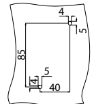
Tamaño de instalación del tornillo
