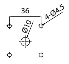
Tamaño de instalación del panel principal
